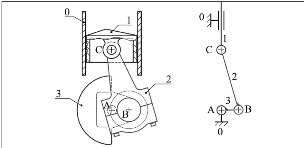
Рис. 3. Статическая конструктивная схема узла—цилиндр—поршень—шатун—коленчатый вал двигателя внутреннего сгорания
