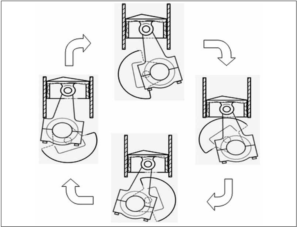
Рис. 4. Фрагменты динамической конструкционной схемы узла цилиндр-поршень-шатун-коленчатый вал двигателя внутреннего сгорания
