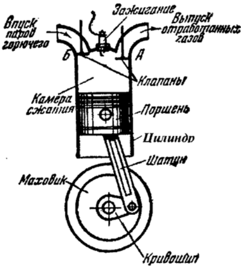
Рис. 1. Конструкционная схема поршневого двигателя внутреннего сгорания
